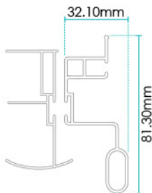
Door Handle
